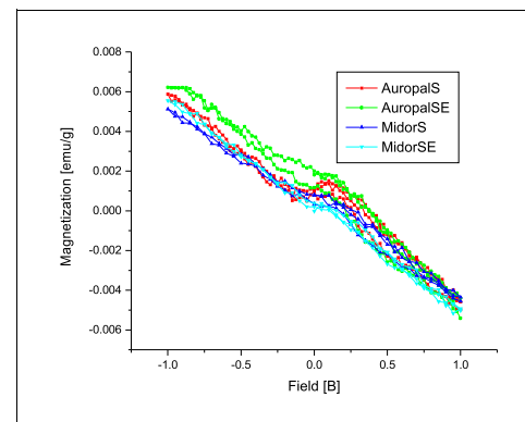
Slika 2: Krivulje magnetjenja [B/H] za dentalne zlitine Zlatarne Celje, d.d.
