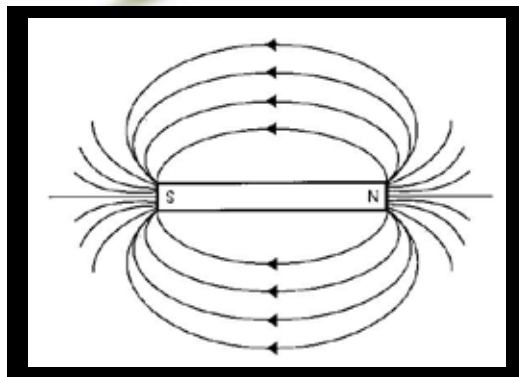
Slika 1: Magnetno polje
